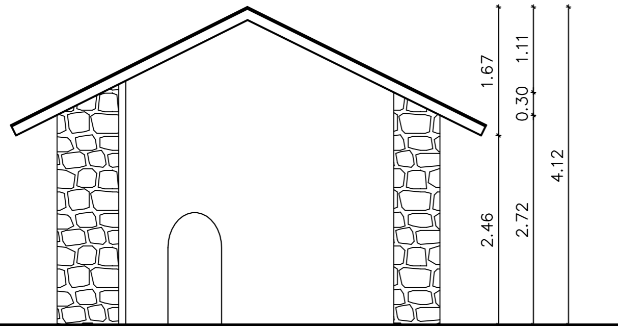
ΤΟΜΗ 1-1 ΜΠΑΡΟΥΤΟΜΥΛΟΥ
