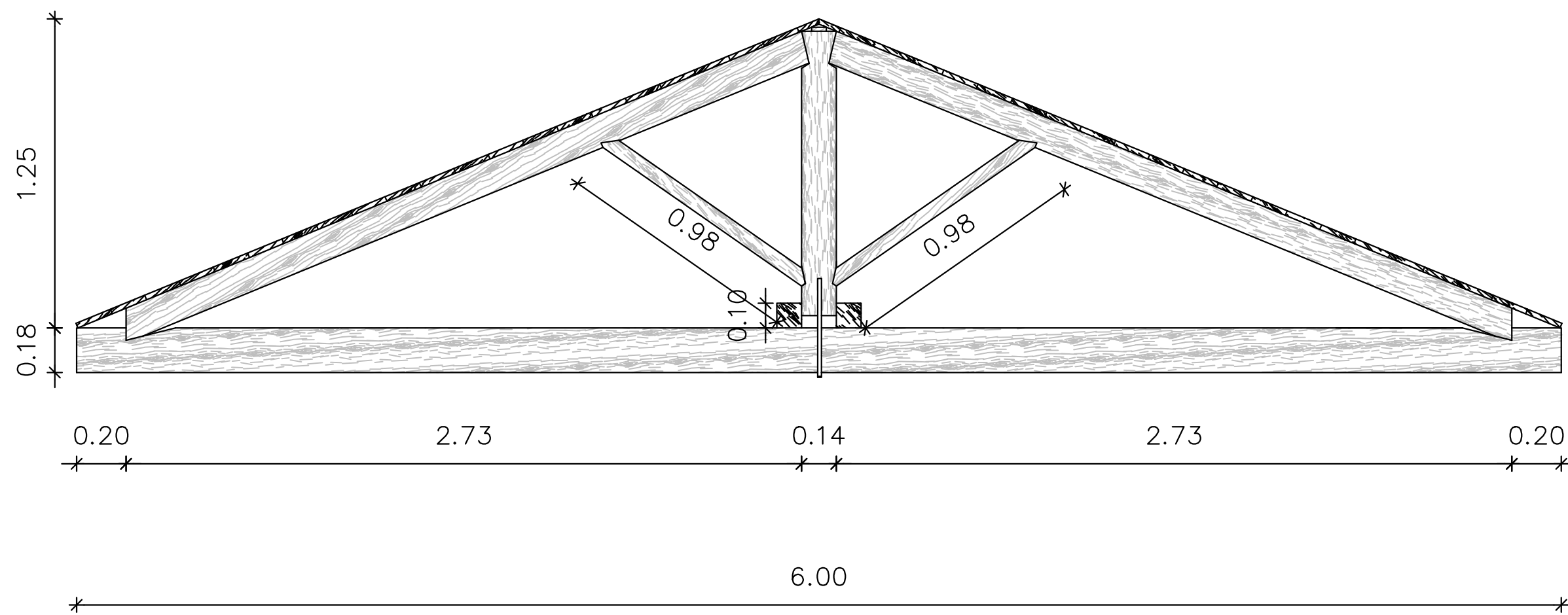
ΛΕΠΤΟΜΕΡΕΙΑ ΞΥΛΙΝΟΥ ΖΕΥΚΤΟΥ
