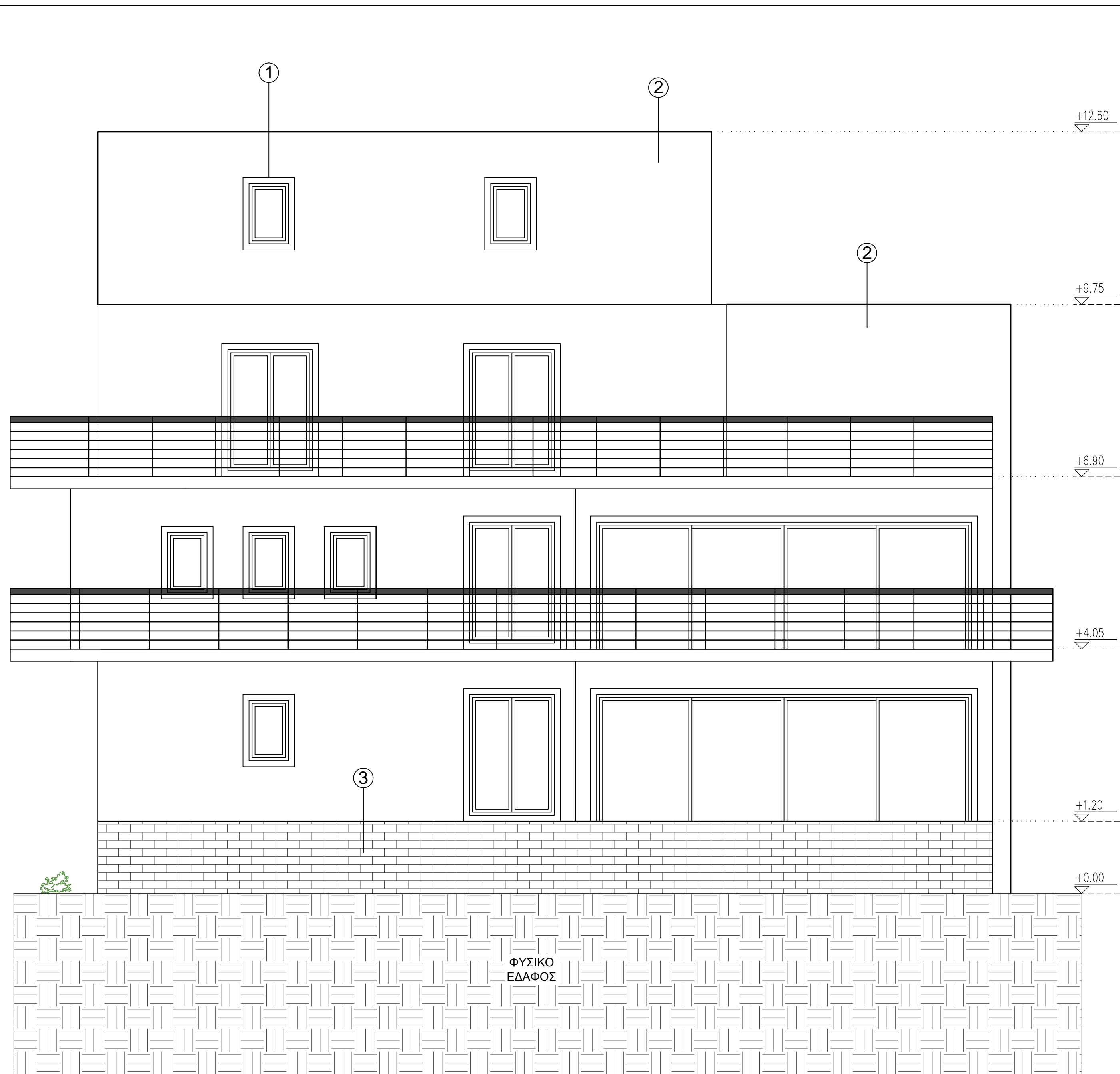
Κύρια Όψη / Κλίμακα 1:50
