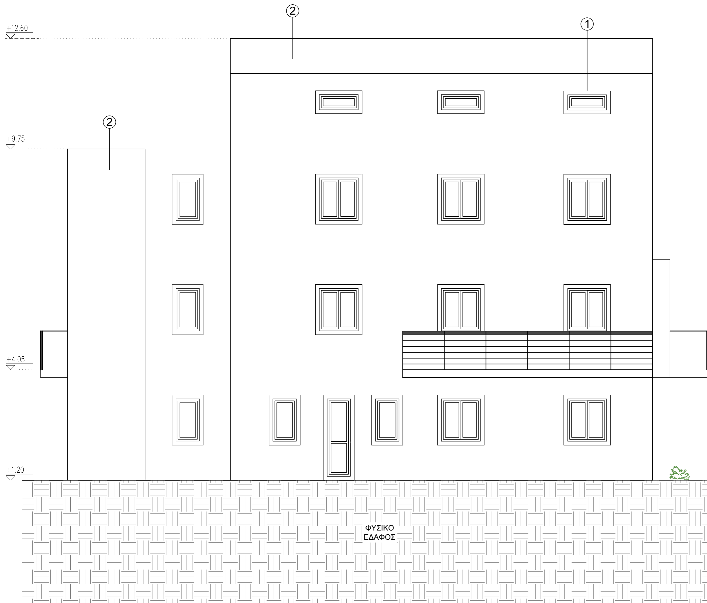
Οπίσθια Όψη / Κλίμακα 1:50
