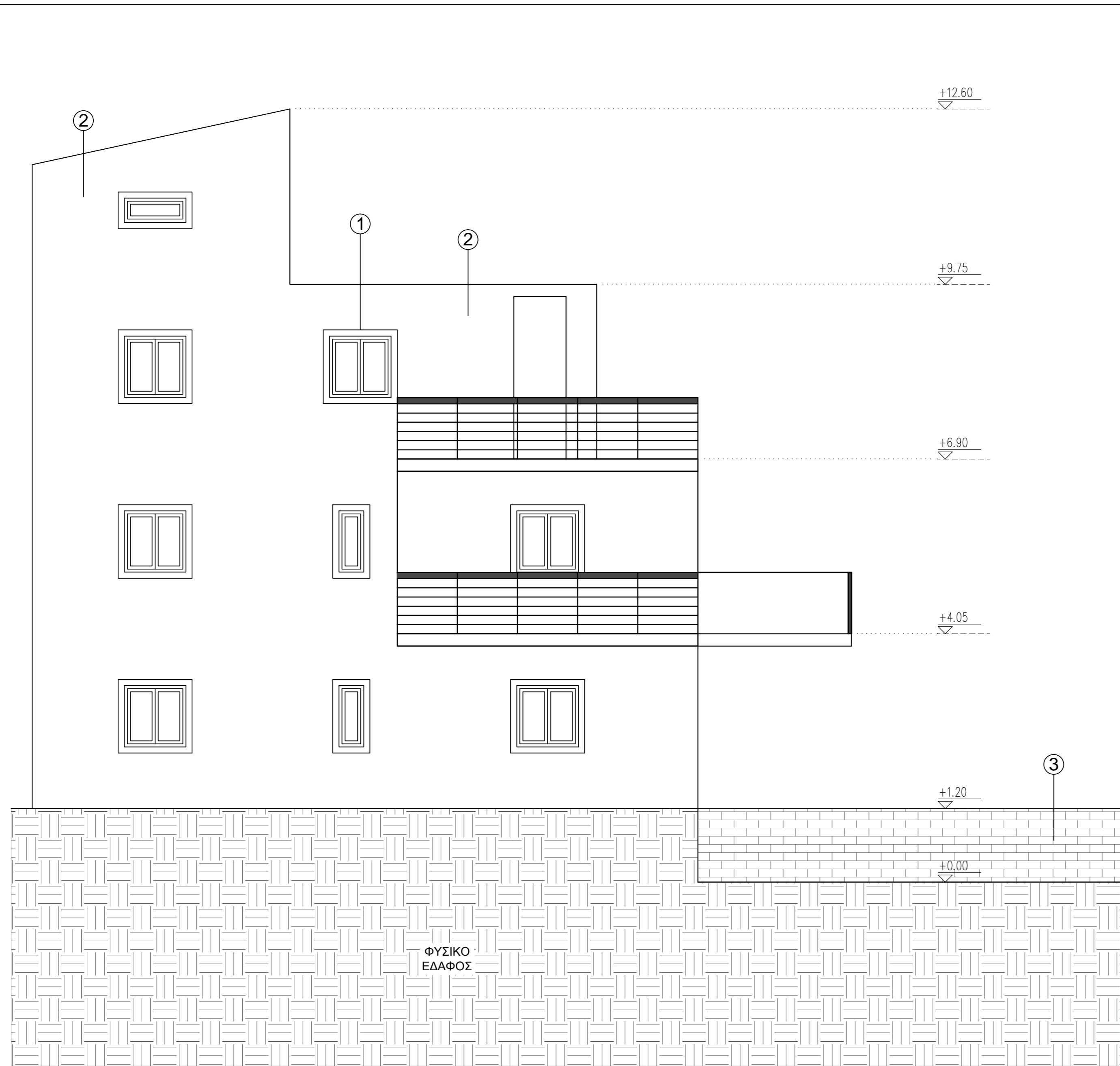
Ανατολική Όψη / Κλίμακα 1:50
