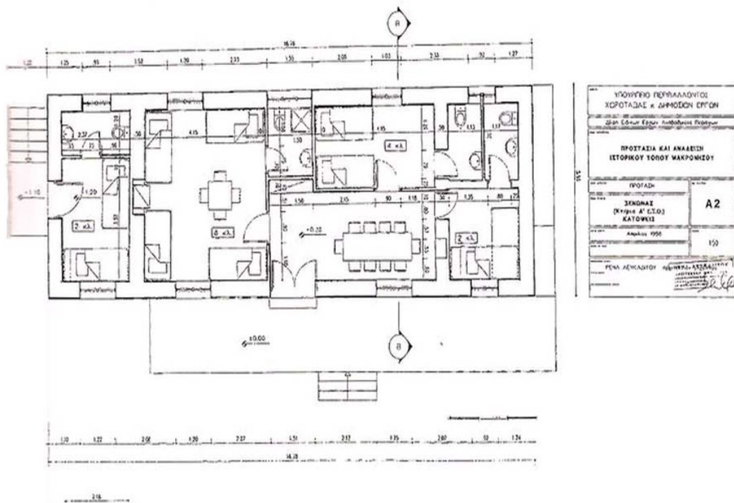
Εικόνα 51 η : Αρχιτεκτονική Κάτοψη αναψυκτηρίου. Μελέτη αποκατάστασης και λειτουργία ως Ξενώνας (ΥΠΕΧΩΔΕ Απρίλιος 1996).
