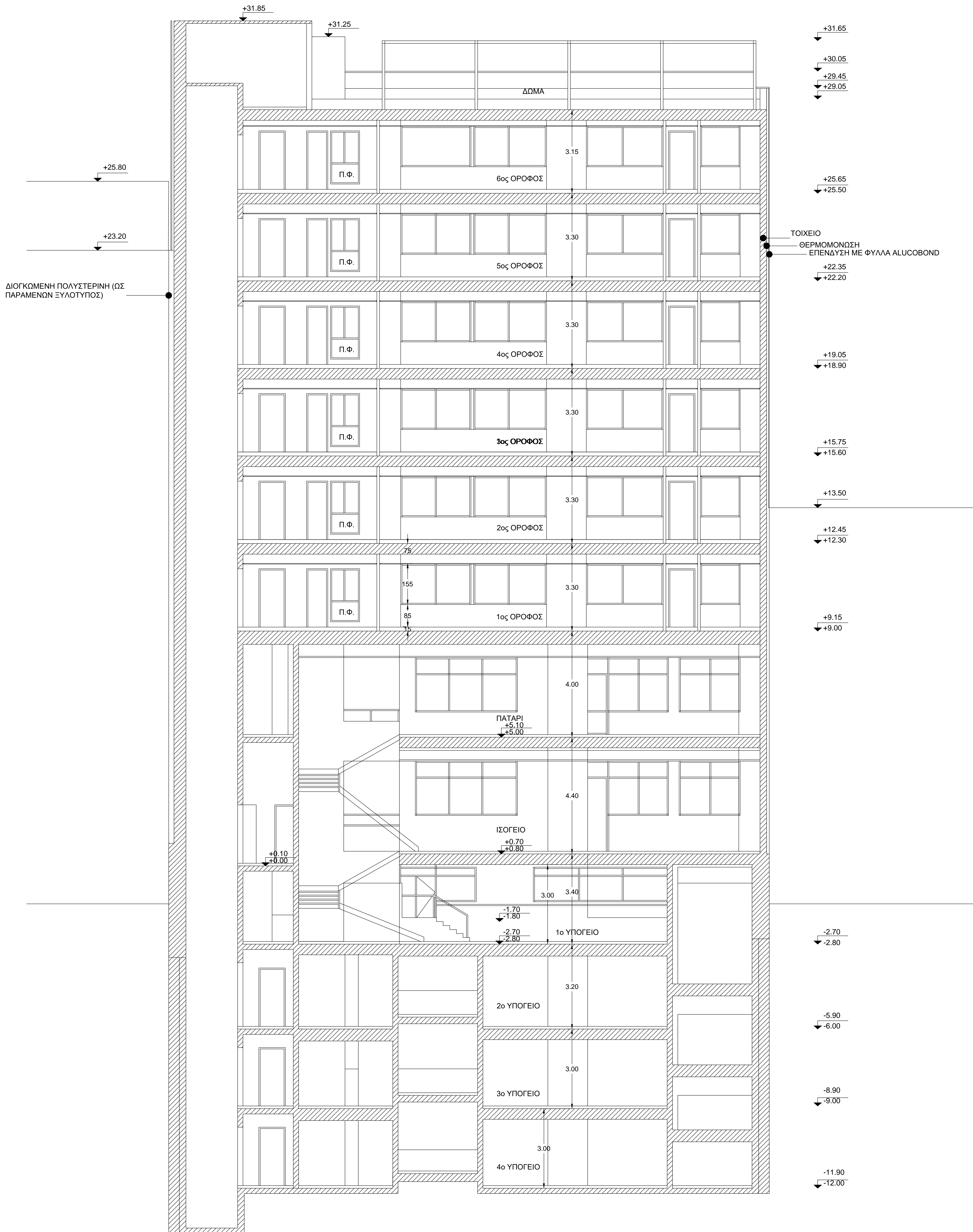
ΤΟΜΗ 2-2
