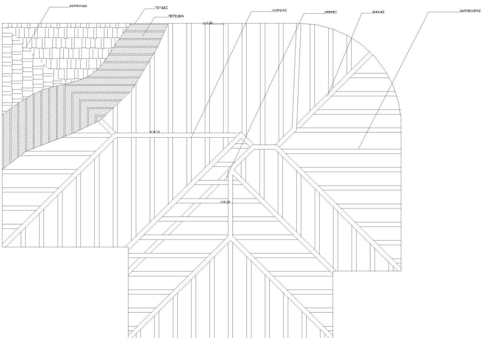
Κάτοψη φέροντα οργανισμού στέγης
