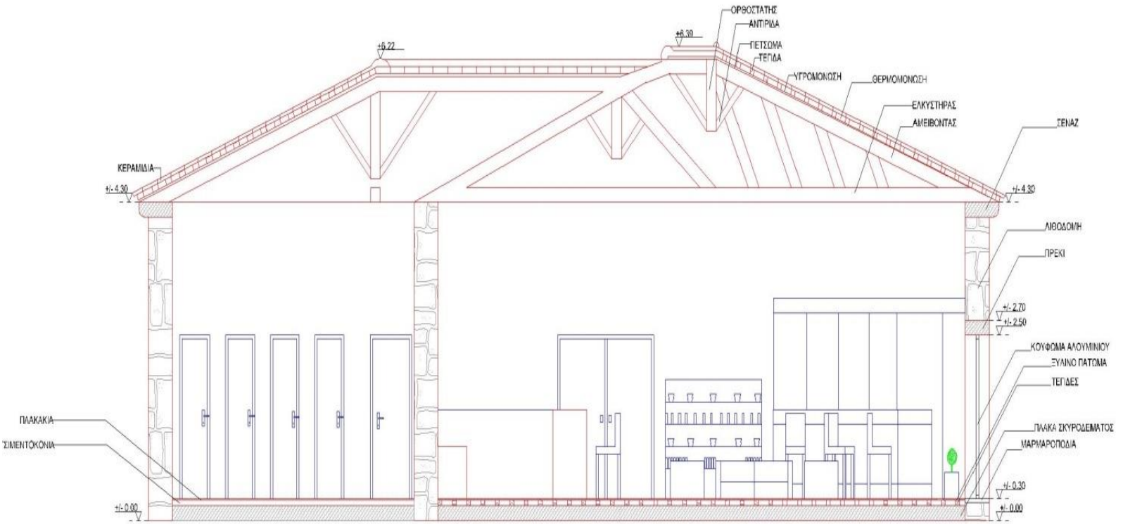
Τομή Α-Α
