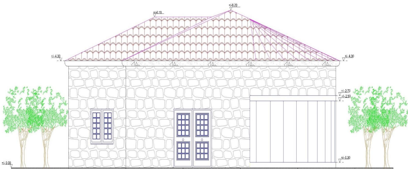
Πλάγια δεξιά όψη
