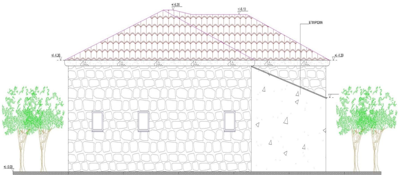
Πλάγια αριστερή όψη
