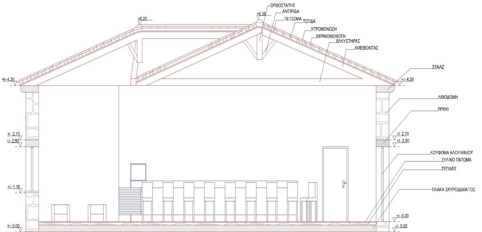
Τομή Β-Β
