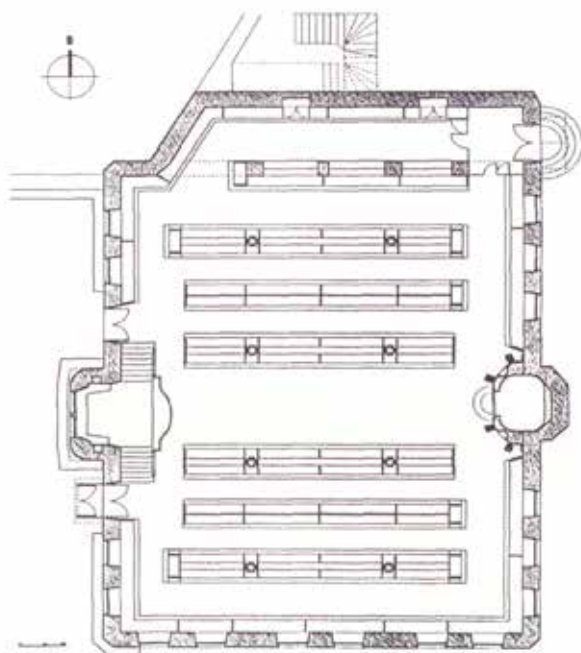
Εικ. 20: Η κάτοψη της Συναγωγής Kahal Kadosh Yashan.
